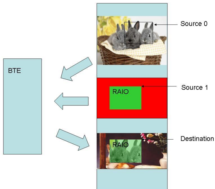
圖 13-27 : 16bpp Pixel Mode Hardware Data Flow
