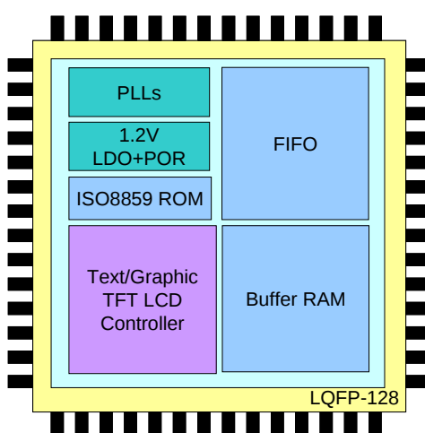
圖 1-2 : Chip Diagram
