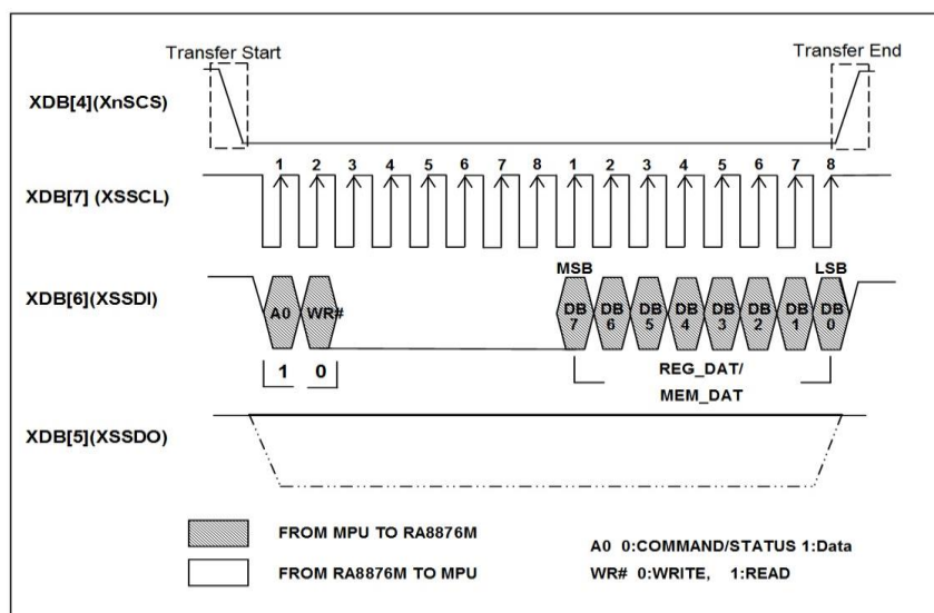
圖 7-14 : Data Write on 4-Wire SPI-Bus
