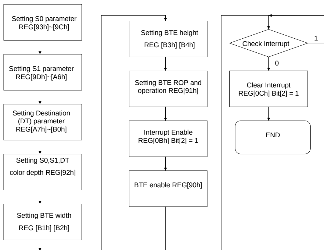
圖 13-9 : Flow Chart – Check Int
