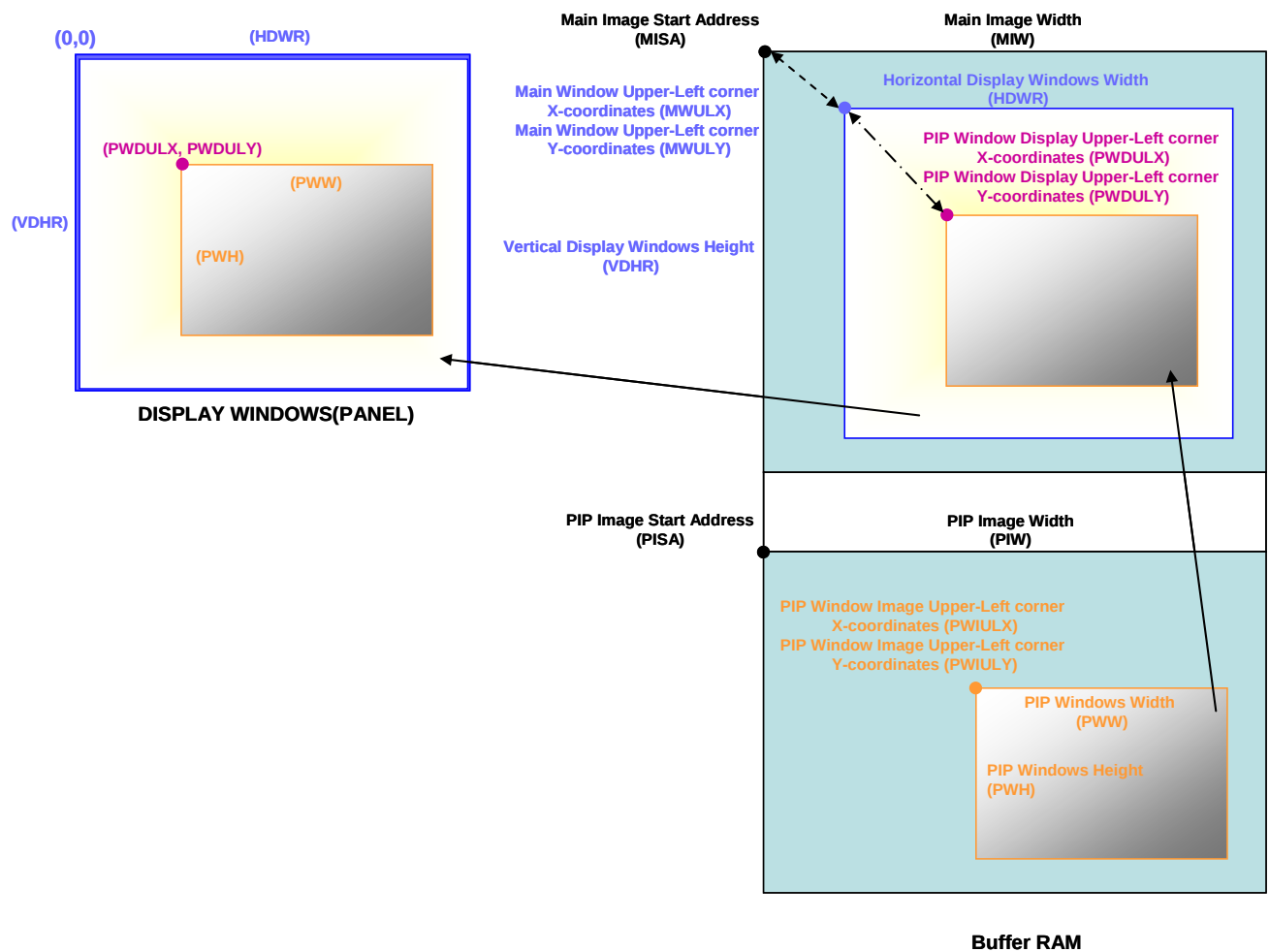
圖 19-2 : LCD Display
