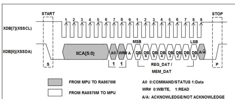
圖 7-21 : Data Read on IIC-Bus
