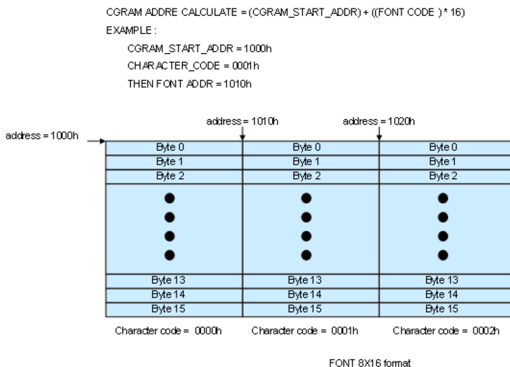
圖 14-4 : Font 8X16 Array in Buffer RAM
