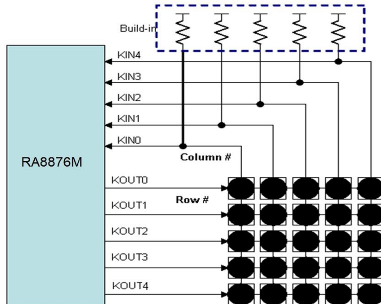
圖 17-1 : Key-Pad Application
