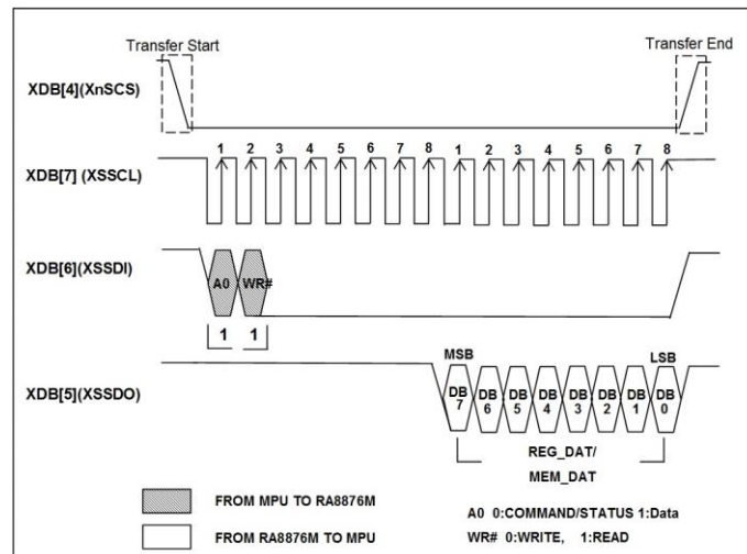
圖 7-15 : Data Read on 4-Wire SPI-Bus
