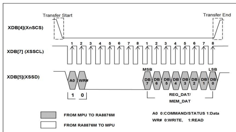
圖 7-11 : Data Write on 3-Wire SPI-Bus
