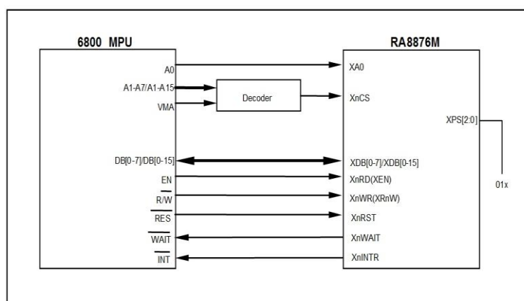
圖 7-2 : 6800 MPU Interface
