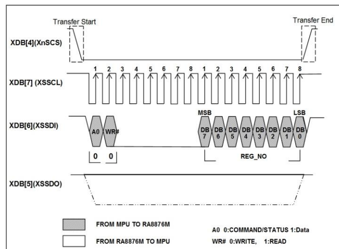
圖 7-16 : CMD Write on 4-Wire SPI-Bus
