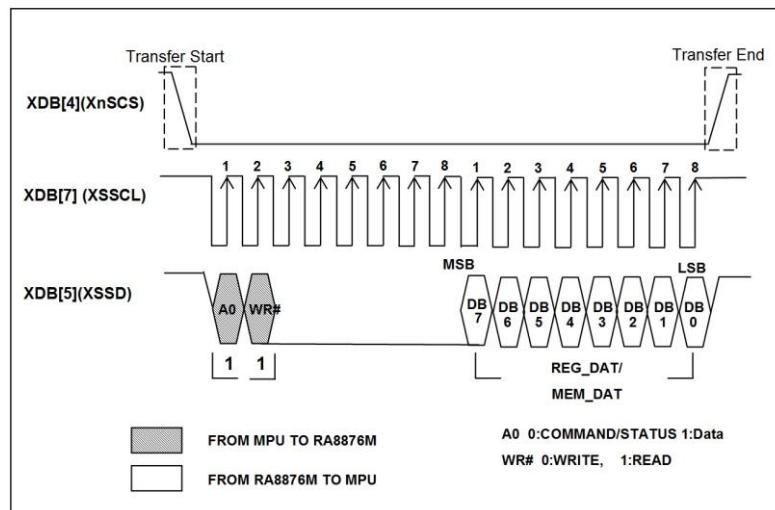
圖 7-10 : Data Read on 3-Wire SPI-Bus
