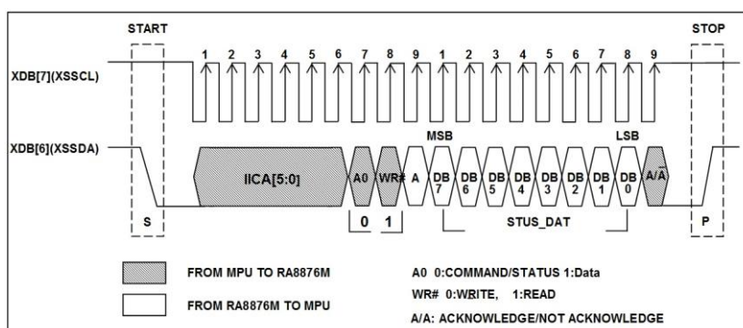
圖 7-22 : CMD Write on IIC-Bus
