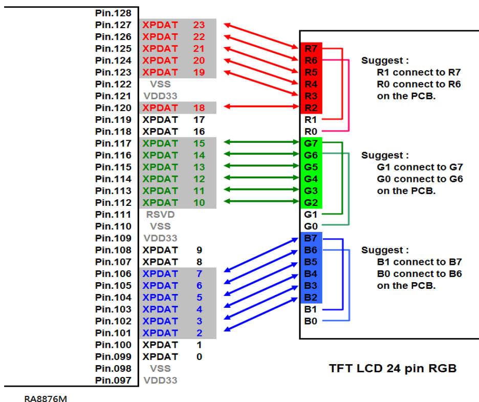
Figure 10-2 : RA8876M 色深 18bit 腳位與 LCD 螢幕腳位對應
