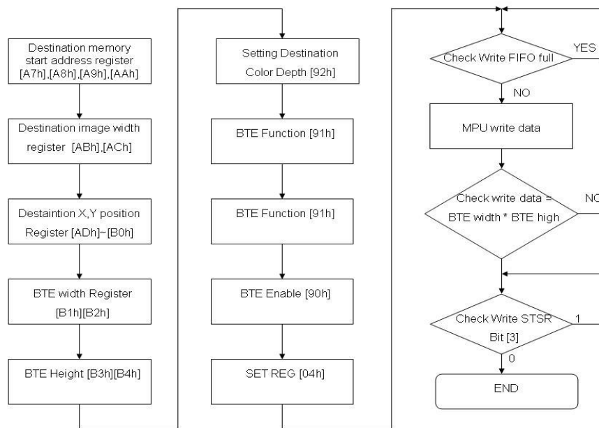
圖 13-20 : Flow Chart
