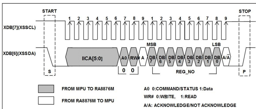
圖 7-22 : CMD Write on IIC-Bus
