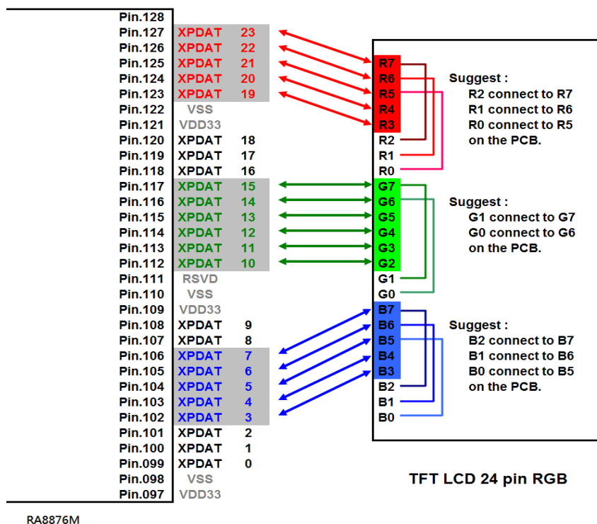
Figure 10-3 : RA8876M 色深 16bit 腳位與 LCD 螢幕腳位對應
