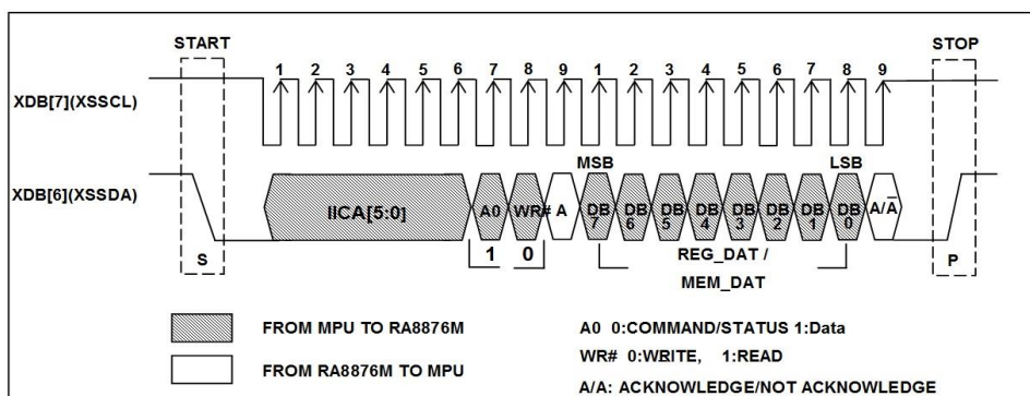
圖 7-20 : Data Write on IIC-Bus
