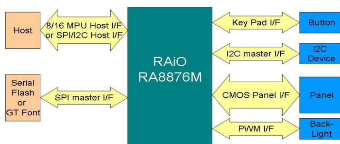
圖 1-1 : System Diagram
