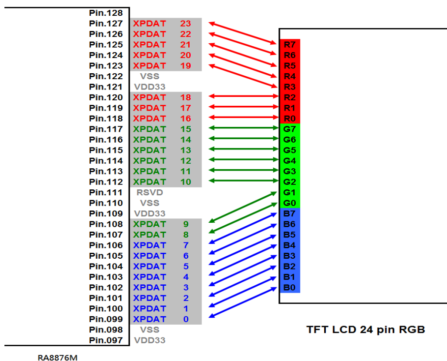
Figure 10-1 : RA8876M 色深 24bit 腳位與 LCD 螢幕腳位對應
