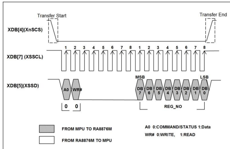
圖 7-9 : CMD Write on 3-Wire SPI-Bus
