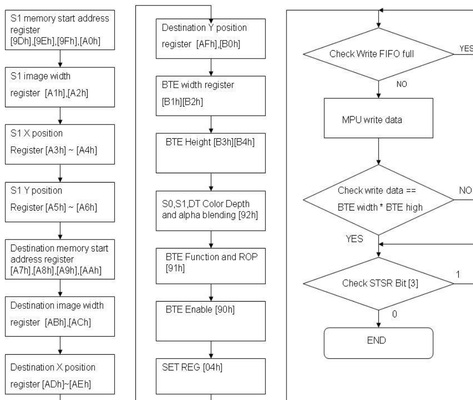
圖 13-6 : Flow Chart
