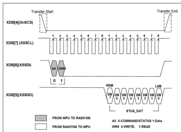
圖 7-17 : Status Read on 4-Wire SPI-Bus
