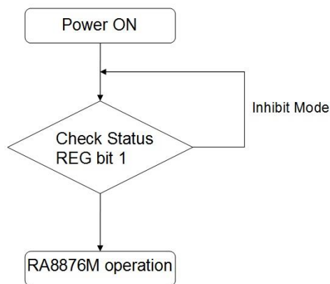
Figure 6-4： 開機後使用 RA8876M 必須先檢查 Status REG bit 1 狀態
