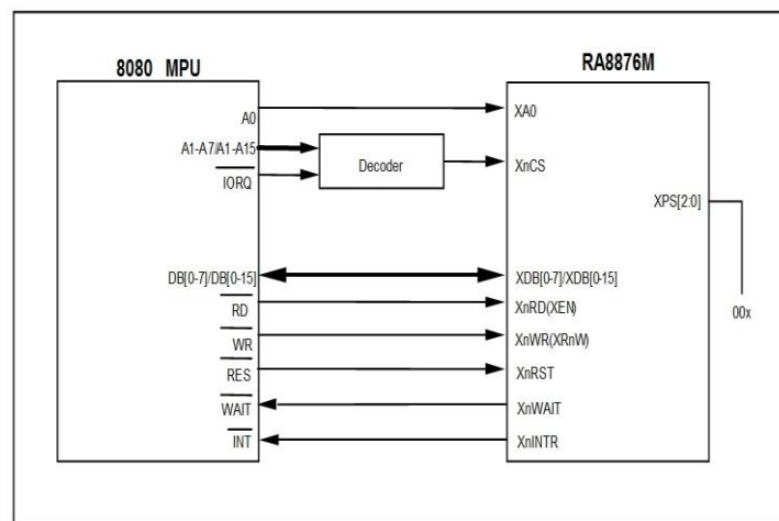
圖 7-1 : 8080 MPU Interface
